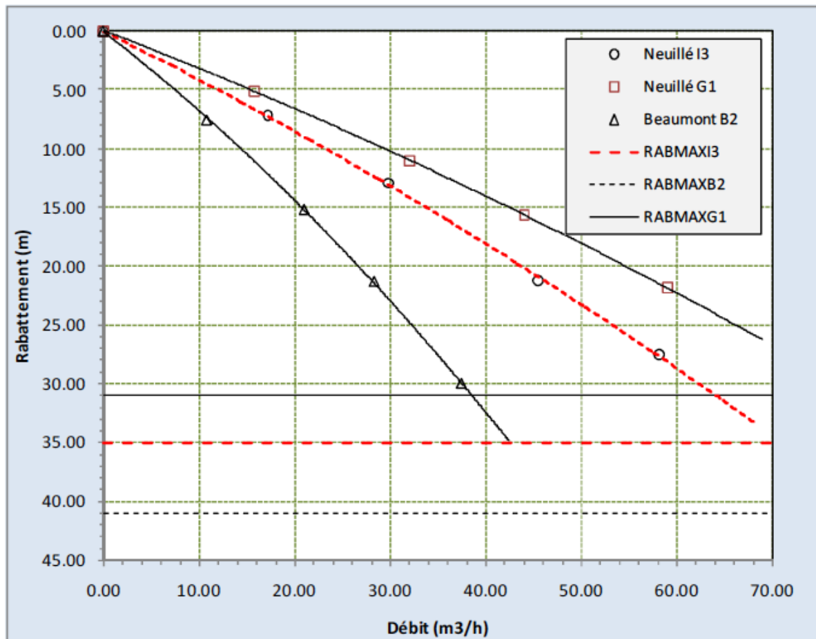
Figure 5 : Productivités comparées des forages d'essai de Beaumont-la-Ronce (B2) et de Neuillé-Pont-Pierre (G1 et I3)
